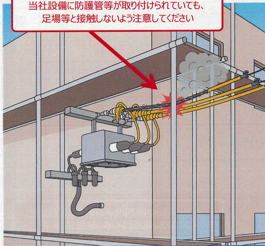
足場に接触して火災が発生した事例
